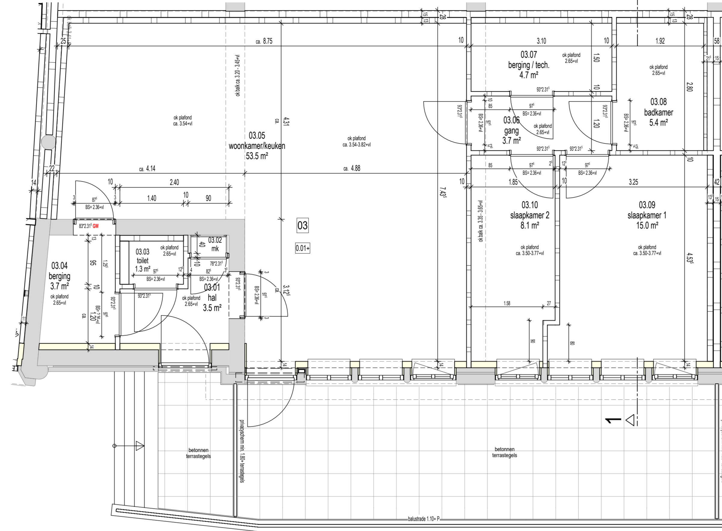
Plattegrond - Afbouw -
