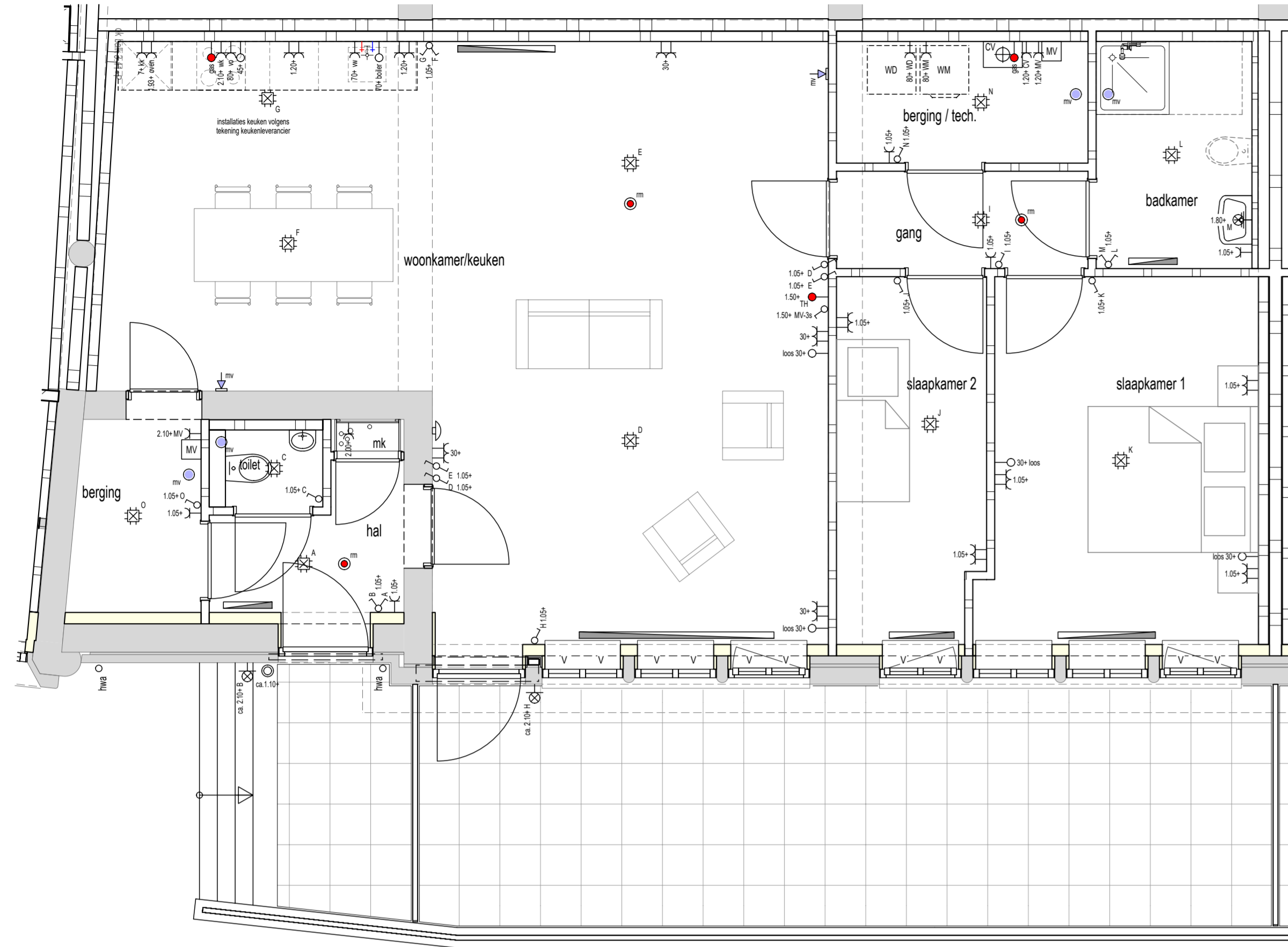
Plattegrond - Installaties -
