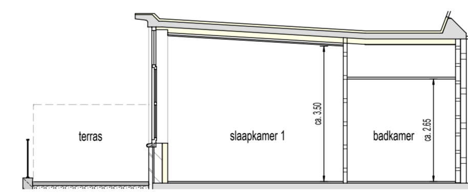
Doorsnede 1-1
