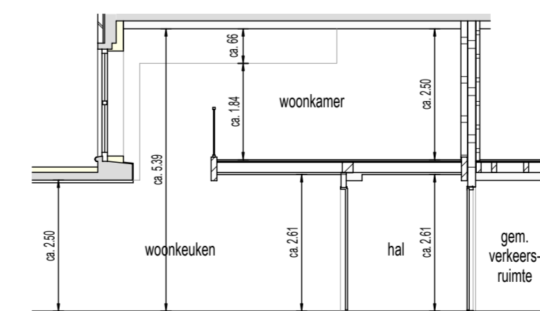
Doorsnede 2-2
