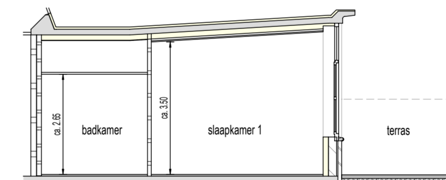
Doorsnede 1-1
