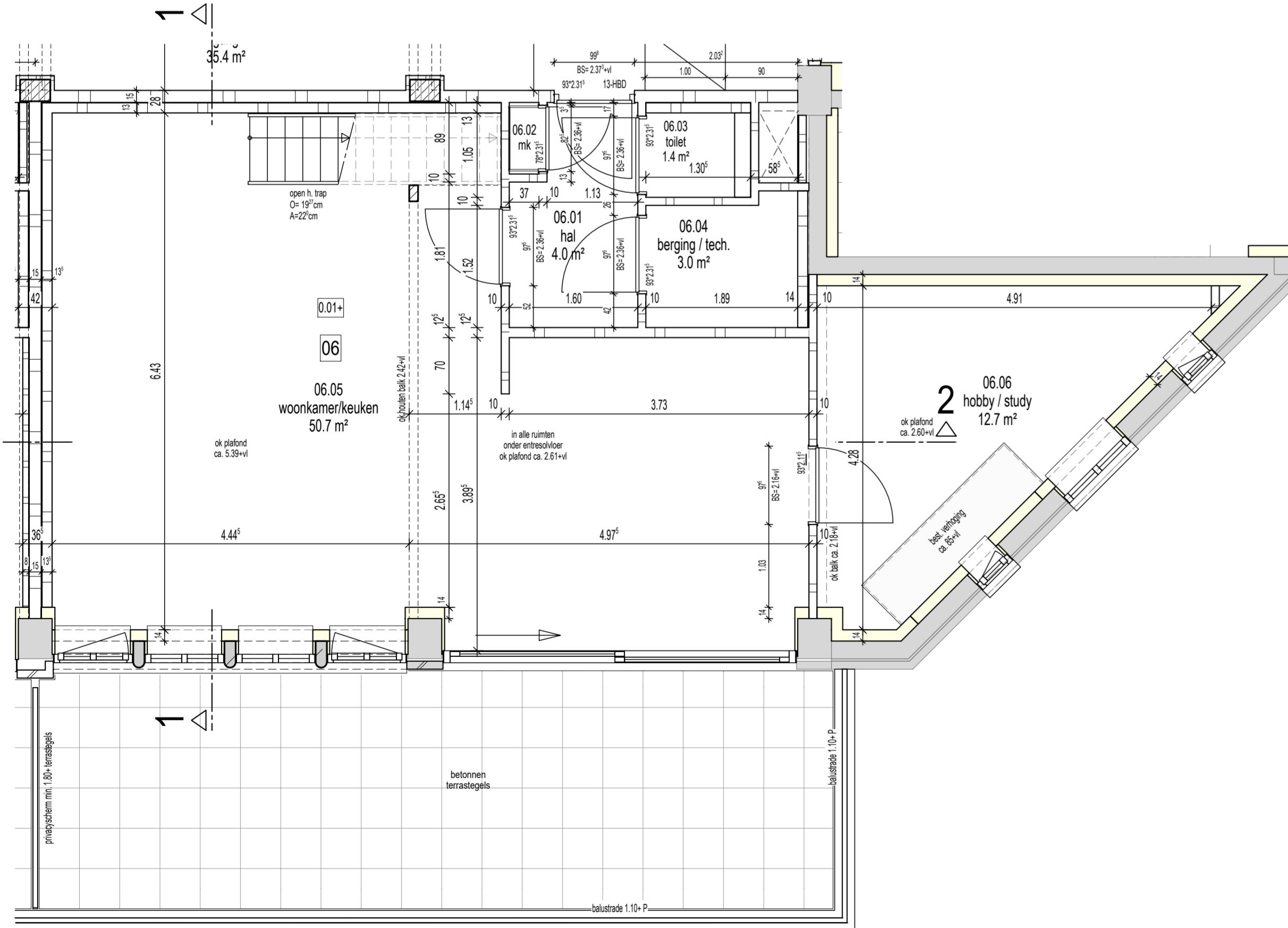
Begane grond - Afbouw -
