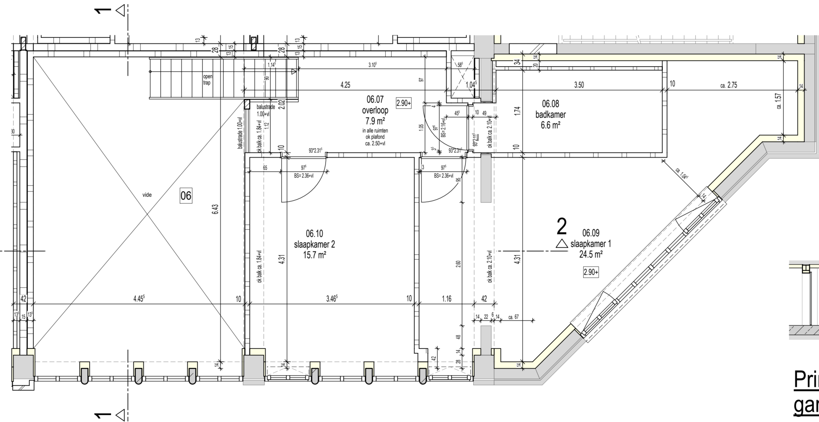
Eerste verdieping - Afbouw -
