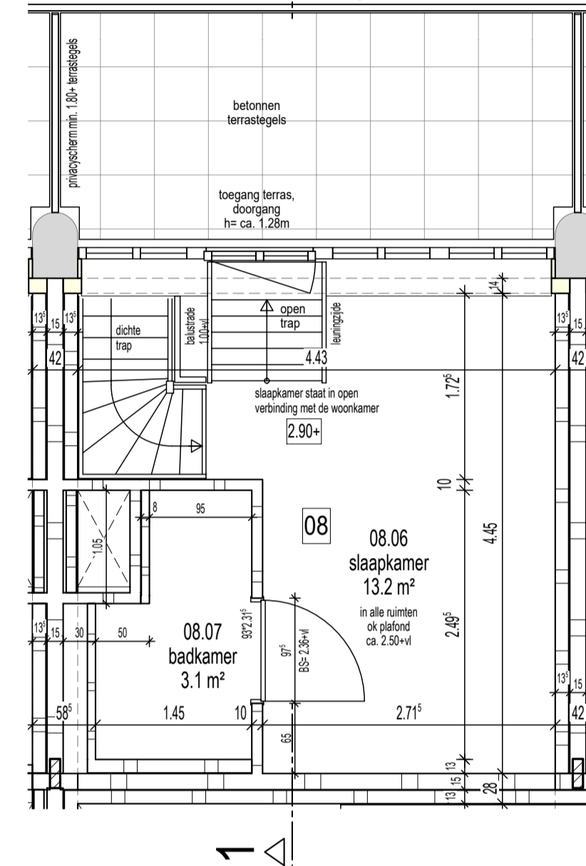
Eerste verdieping - Afbouw -
