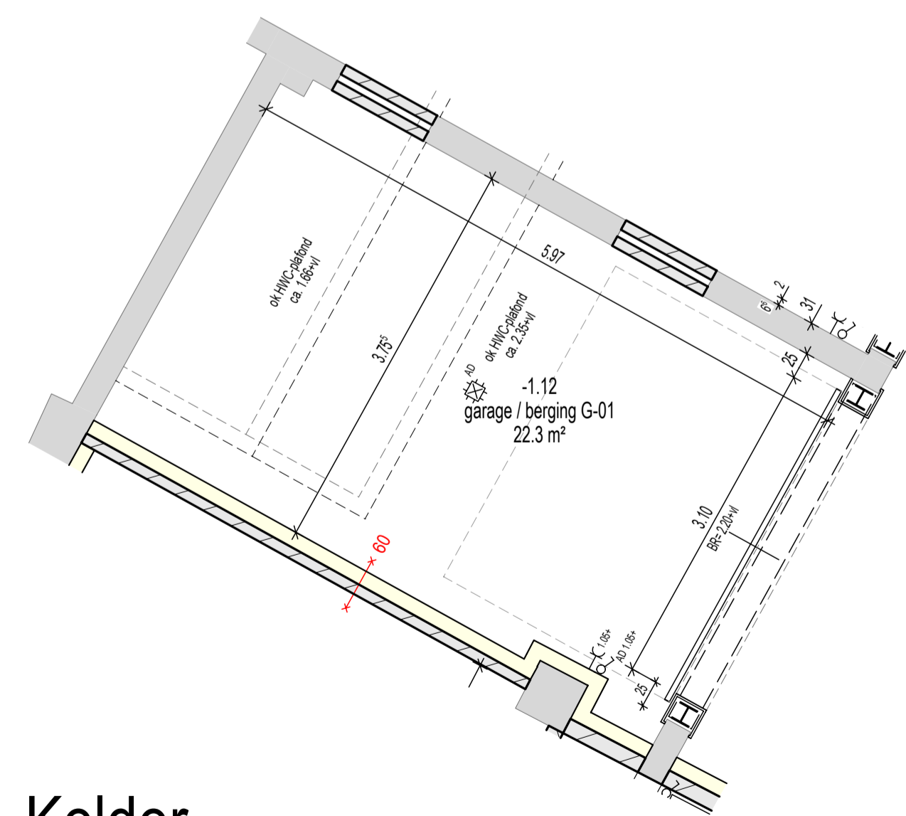
Kelder - Installaties + Afbouw -
