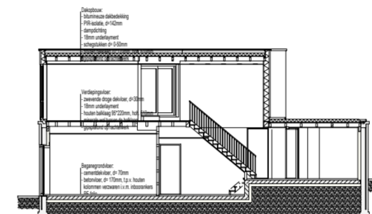
Doorsnede H-H
