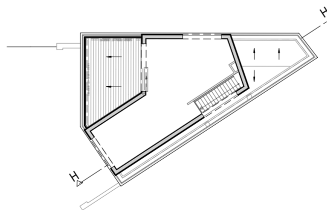
Plattegrond Eerste verdieping
