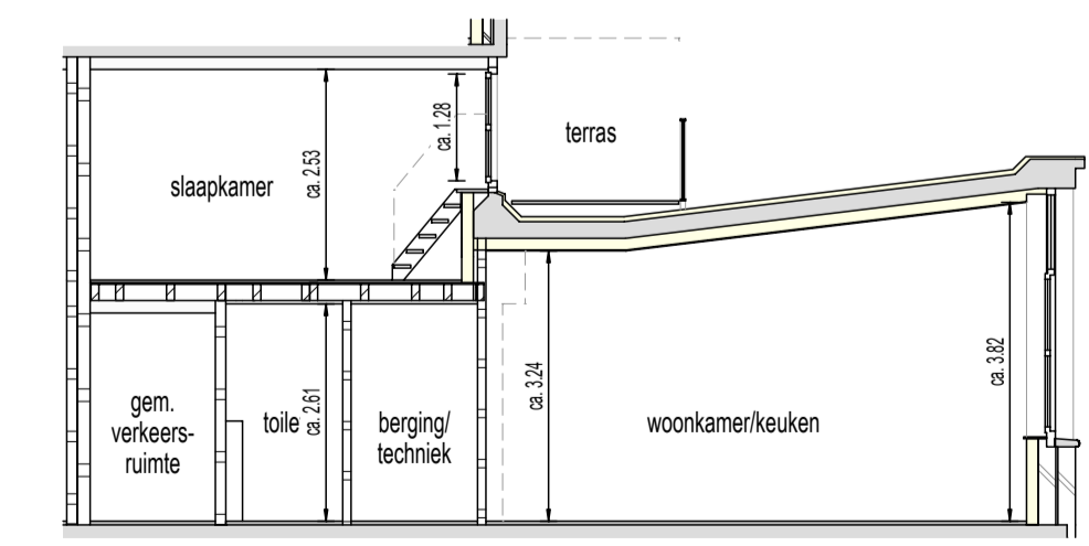
Doorsnede 1-1
